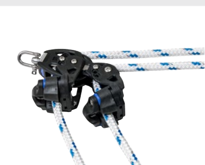
Tandemblock för ändlös manöverlina. PBB50 Art. nr. 405-001-40R (max Ø10 mm lina) PBB60 Art. nr. 406-001-40R (Ø12 mm lina)
